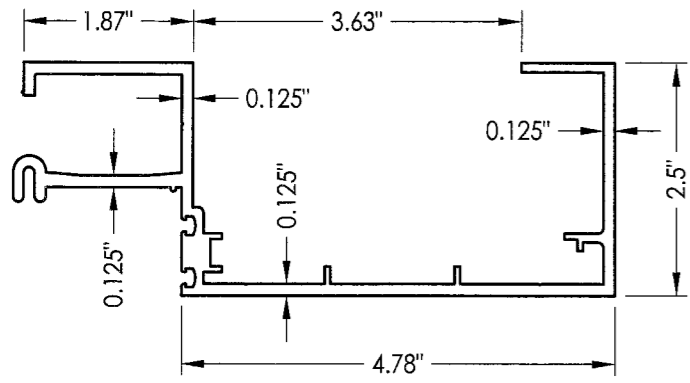
1 JAMB
